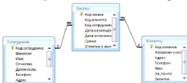
Рис. 2. Схема данных
