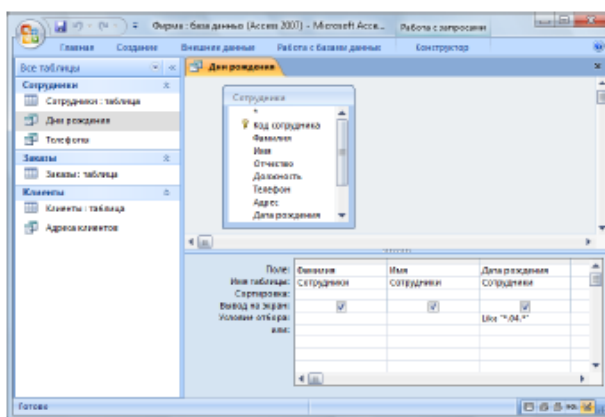
Рис. 5. Создание запроса
