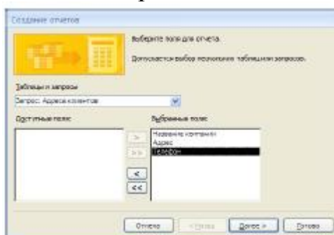
Рис. 15. Мастер отчетов
