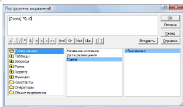
Рис. 8. Построитель выражений
